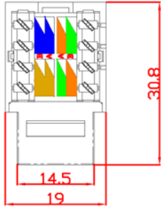
Cat.5e Keystone
