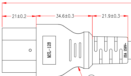
IEC 320 C21(MSL-128)
