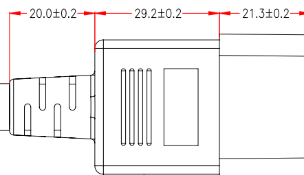
IEC 320 C20(MSL-120)
