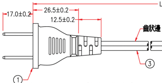
NEMA 1-15P (MSL-101P)
