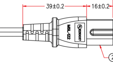
IEC320 C7 (MSL-122)
